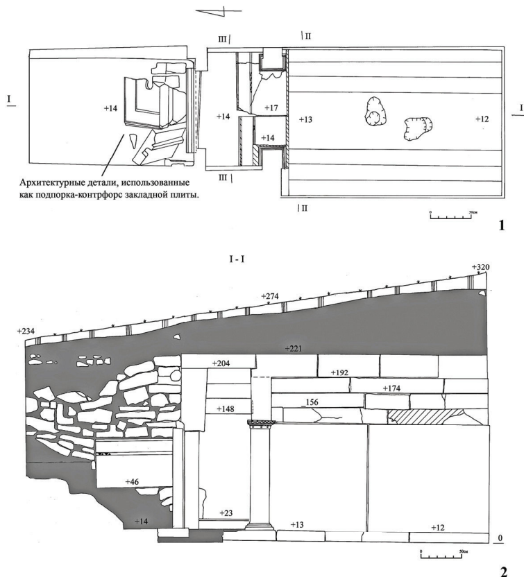
Рис. 1. Уступчатый склеп. 1 – план; 2 – разрез по линии I-I.
